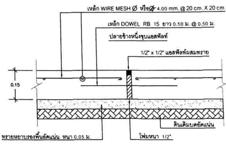
แบบขยาย EXPANSION JOINT ① มาตราส่วน 1:10
