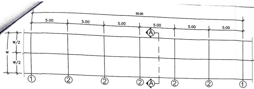
แปลนถนนคอนกรีตเสริมเหล็ก 2 เลน มาตราส่วน 1:200
