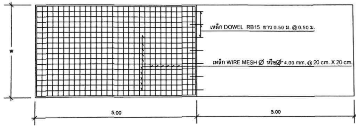
แปลนการเสริมเหล็ก แบบ 1 เส้น มาตราส่วน 1:75
