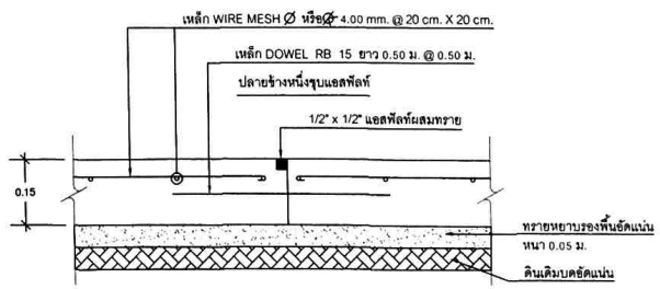
แบบขยาย CONSTRUCTION JOINT ② มาตราส่วน 1:10
