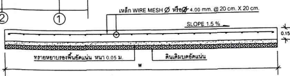
รูปตัด A - A มาตราส่วน 1:25
