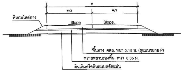
รูปตัดถนนคอนกรีต 2 เลน มาตราส่วน 1:50
