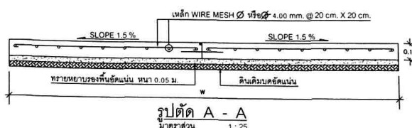
แบบขยาย EXPANSION JOINT ① มาตราส่วน 1:10
