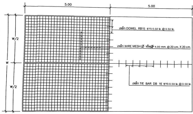
แปลนการเสริมเหล็ก แบบ 2 เลน มาตราส่วน 1:75
