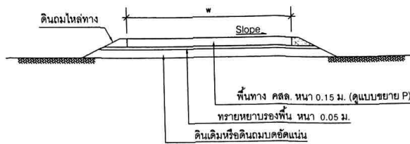
รูปตัดถนนคอนกรีต 1 เลน มาตราส่วน 1:50
